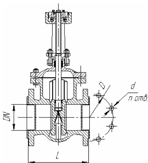
Задвижка параллельная двухдисковая с выдвижным шпинделем
